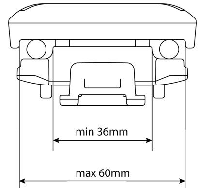
Sattelhalterung
